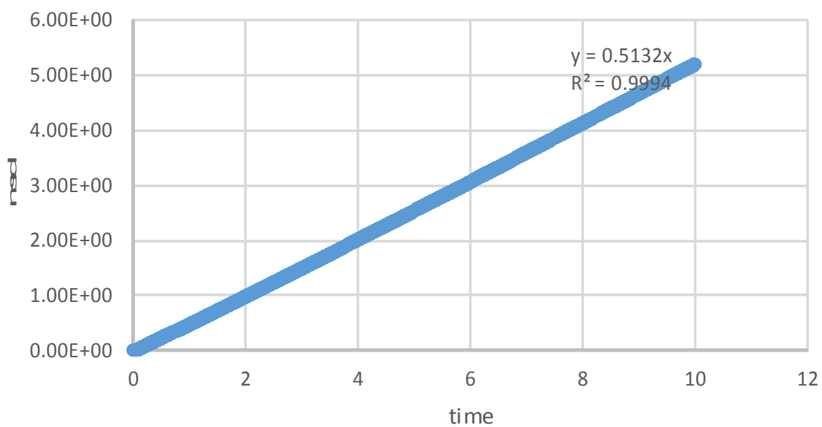
msd liq
