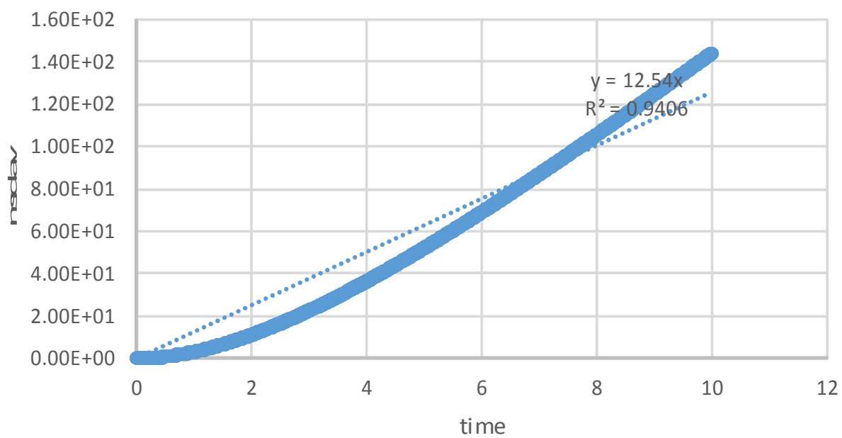
MSD vap
